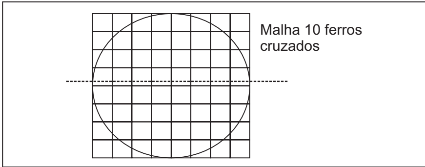
Figura 8 – Estrutura da Malha de Ferro \frac{1}{4} ' do Fundo da Cisterna
