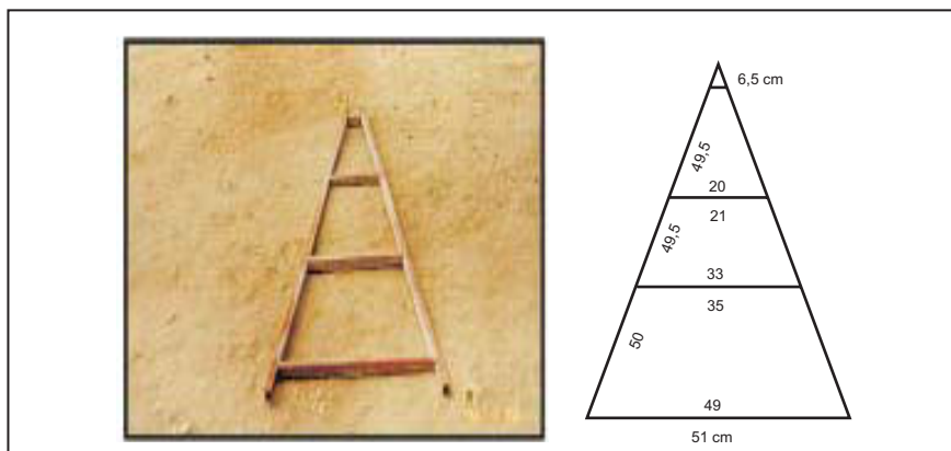
Figura 5 – Foto e Desenho do Gabarito das Placas da Tampa da Cisterna Foto: PRODHAM.
