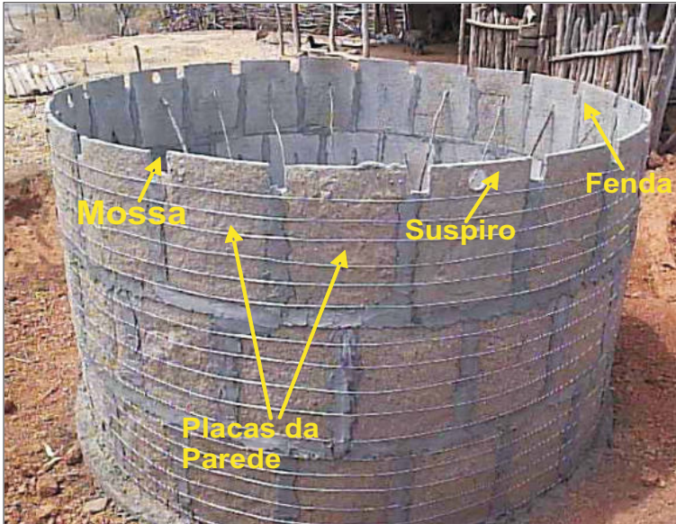
Foto 2 – Detalhes das Placas da Parede da Cisterna
