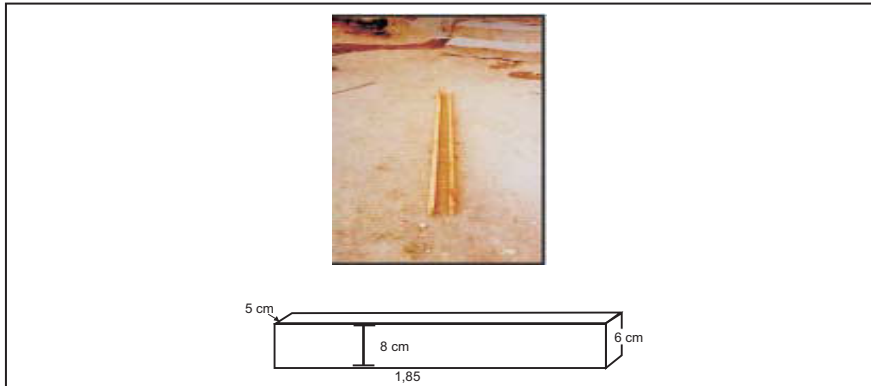
Figura 4 – Foto e Desenho do Gabarito dos Trilhos da Tampa da Cisterna Foto: PRODHAM.
