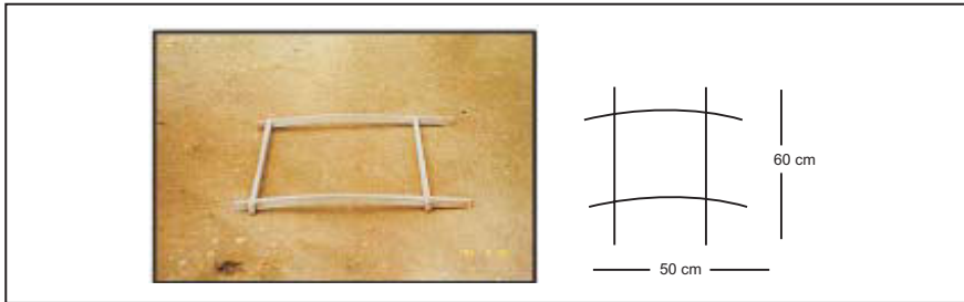
Figura 3 – Foto e Desenho do Gabarito das Placas das Paredes da Cisterna Foto: PRODHAM.
