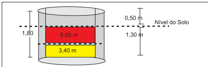
Figura 2 – Dimensões da Escavação
