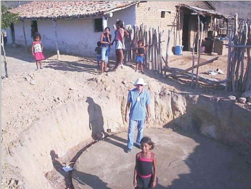
Foto 3 – Aspecto do Piso do Fundo da Cisterna
