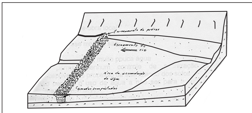
Figura 1 – Barragem Subterrânea Modelo Caatinga
