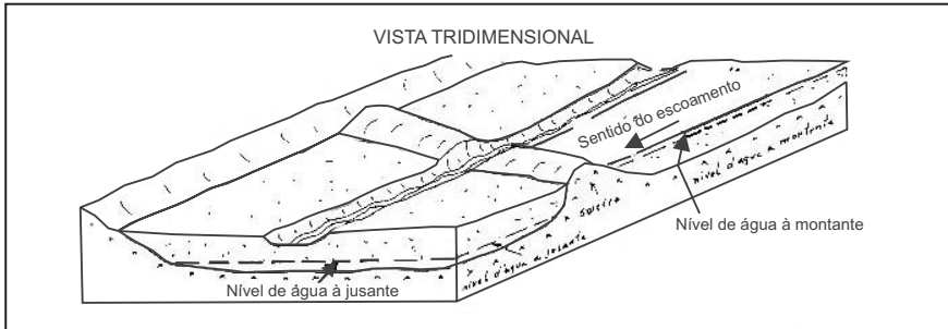
Figura 7 – Barragem Natural por Soleira
