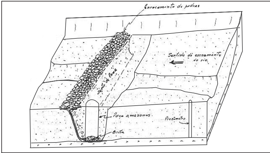
Figura 2 – Barragem Subterrânea Modelo Costa e Melo
