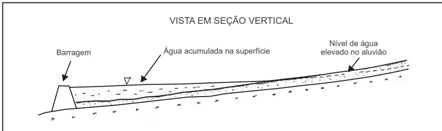
Figura 8 – Barragem Natural por Soleira
