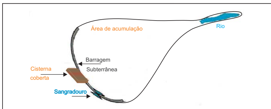
Figura 3 – Barragem Subterrânea Modelo CPATSA
