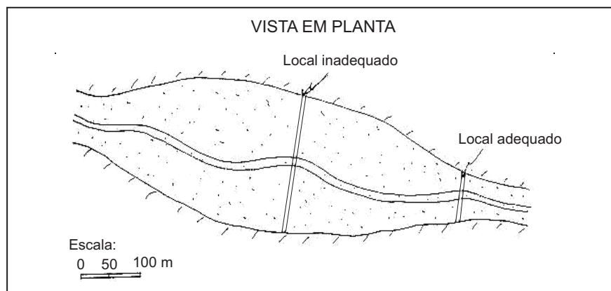
Figura 12 – Localização do Eixo da Barragem
